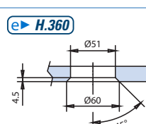
S-FIX-VETRO-60 SV
