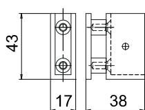
BX-2000-C08 SX • Attacco a vetro sinistro per binario • Left glass connector for track profile • Glashalter links für Laufschiene
