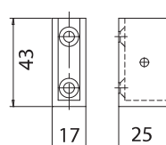
BX-2000-C07 SX • Attacco a parete sinistro per binario • Left wall connector for track profile • Wandhalter links für Laufschiene
