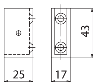
BX-2000-C07 DX • Attacco a parete destro per binario • Right wall connector for track profile • Wandhalter rechts für Laufschiene
