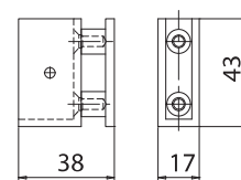
BX-2000-C08 DX • Attacco a vetro destro per binario • Right glass connector for track profile • Glashalter rechts für Laufschiene
